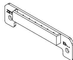
BASETTA PORTAMORSETTI AB84-- VEDI pag. 37.3
